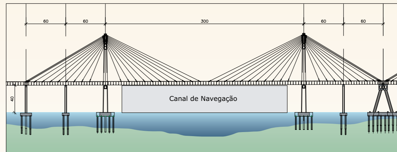
Trecho estaiado lado sul
