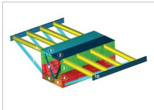
3. Elementos estruturais que compõem a aduela
