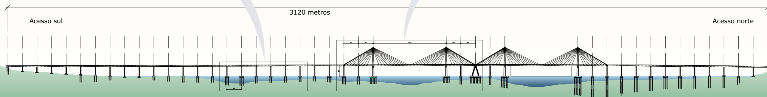
Elevação longitudinal geral
